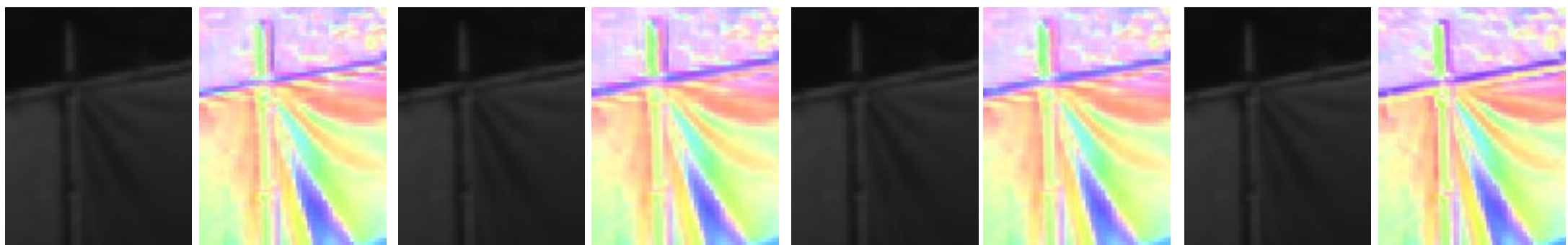
PPID
