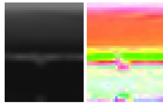
Bicubic
