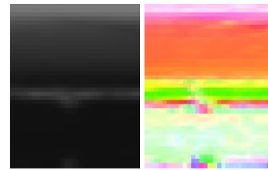
ICPC
