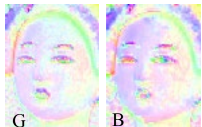
RI | PPID
